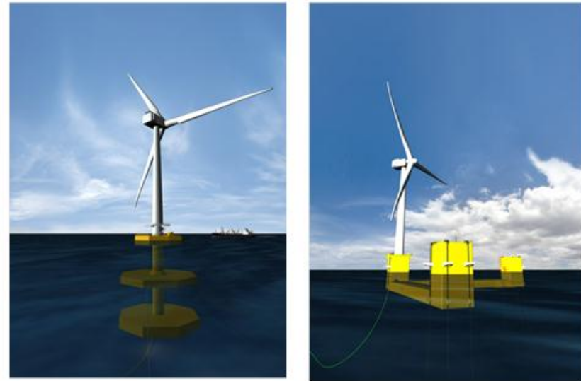
アドバンストスパー浮体 V字型セミサブ浮体
