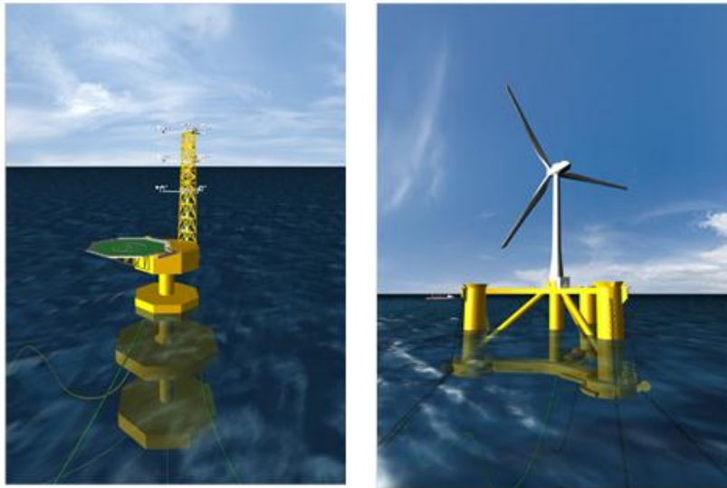
浮体式サブステーション コンパクトセミサブ浮体
