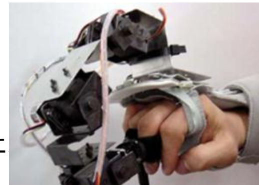
指関節リハビリロボット(プロトタイプ)
